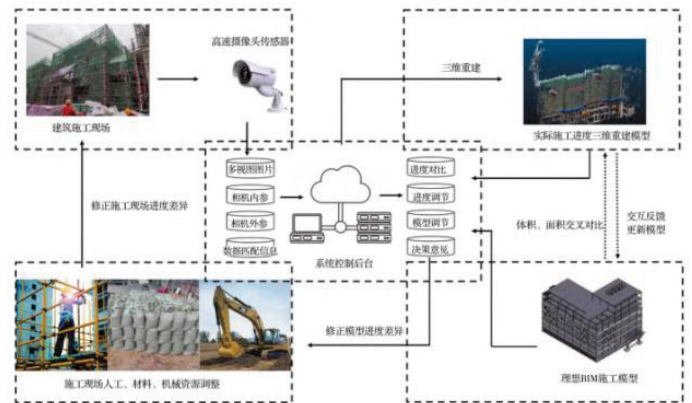
图 1 智慧工地系统结构
